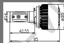
PSX26W, P13
