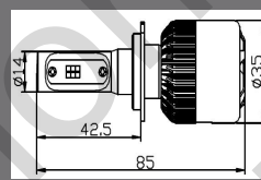
HB1 9004 H/L, HB5 9007 H/L
